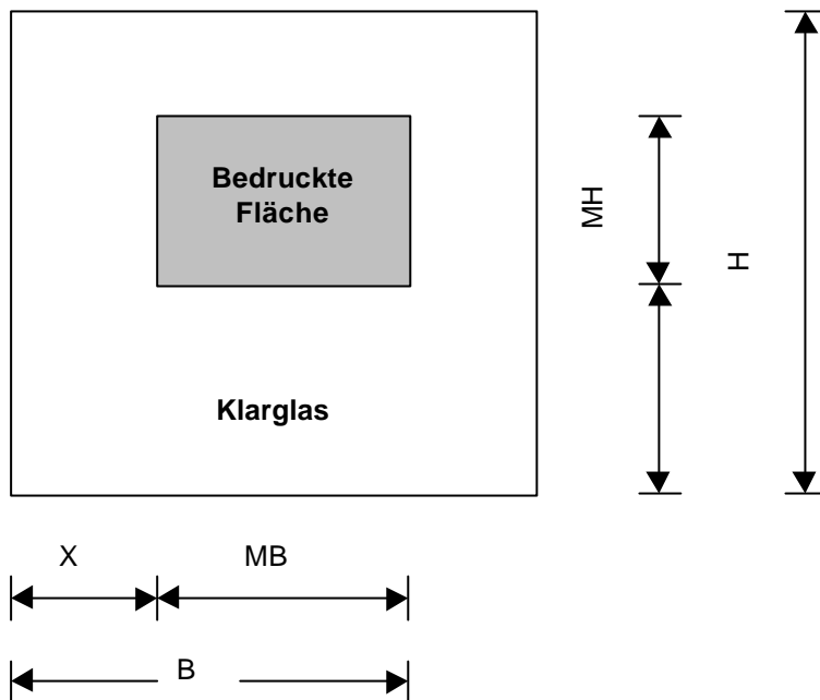
Abbildung 1 zu Tabelle 1 (Toleranz der Abmessung bei Teilemail) und Tabelle 2 (Toleranz der Motivgröße für siebbedruckte Gläser)
